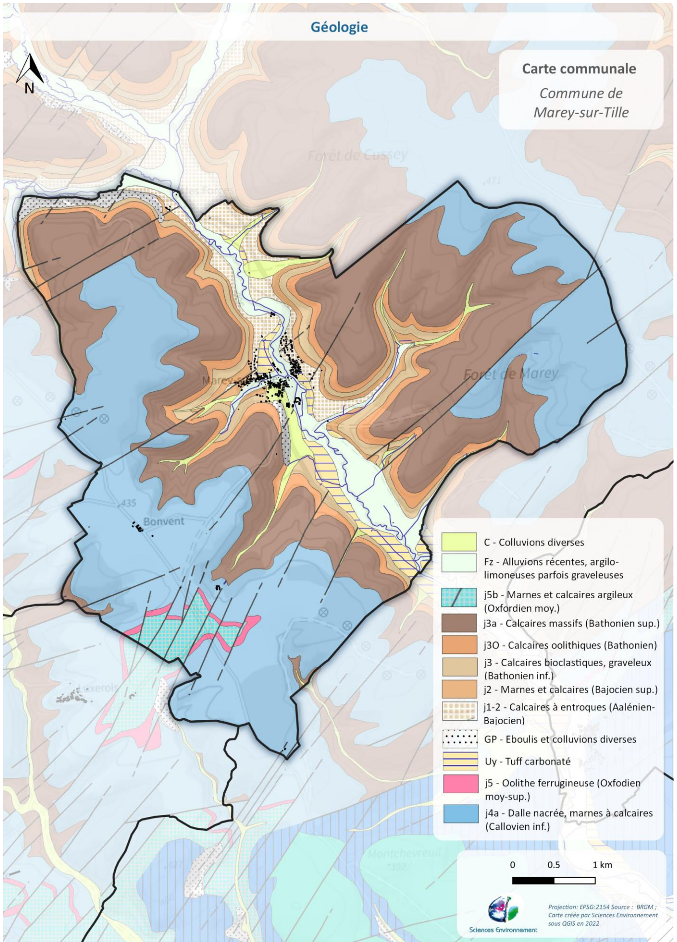
Figure 2 : Géologie
